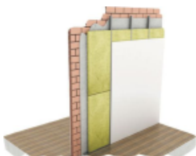
Aïllament façanes
