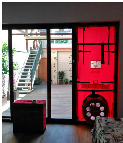
BlowerDoor test
