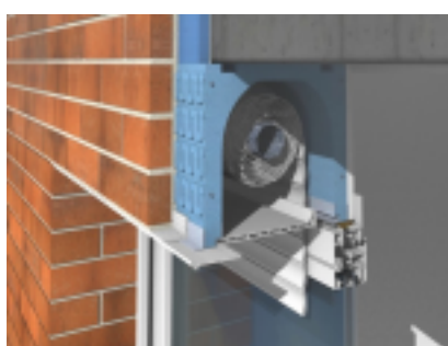
Aïllament caixes de persianes
